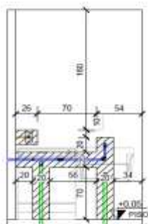
VISTA 1 - ÁREA DE SERVIÇO ESC. 1 : 50
