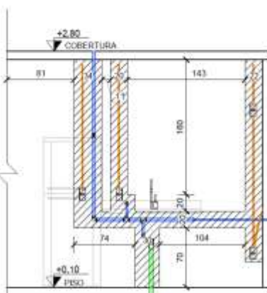
VISTA 1 - COZINHA ESC. 1 : 50
